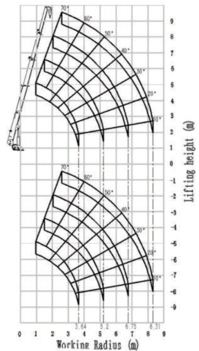
工作范围表 Working Range Diagram
